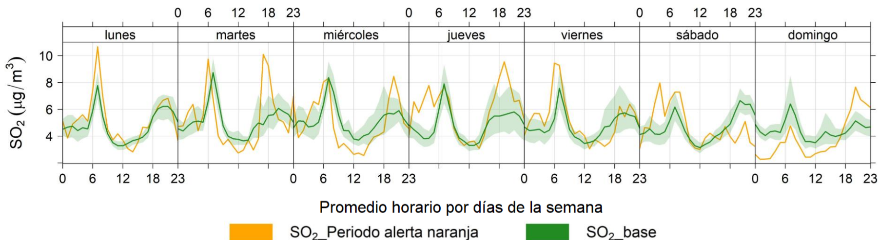
Evolución temporal de concentraciones promedio horarias por días de la semana de SO 2 durante 2023 (SO 2 _base) y su comparativo con el periodo del 3 al 9 de mayo de 2023
