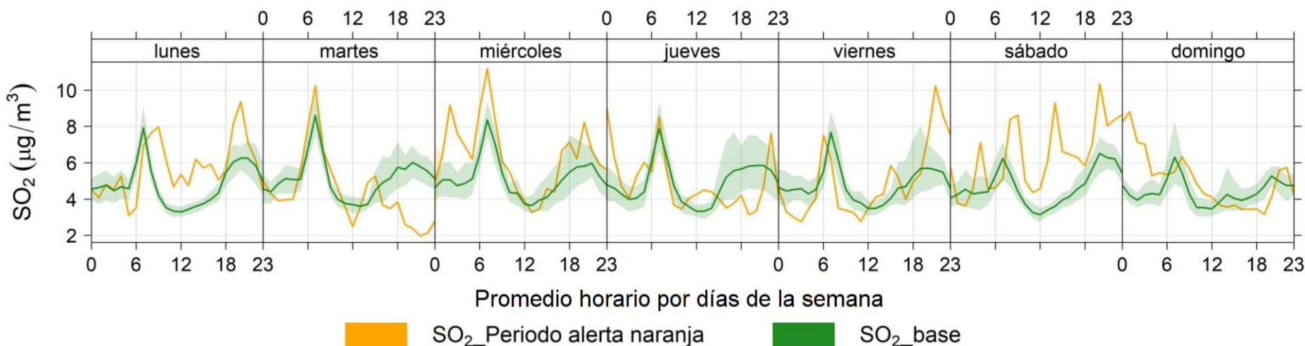
Evolución temporal de concentraciones promedio horarias por días de la semana de SO 2 durante 2023 (SO 2 _base) y su comparativo con el periodo del 10 al 16 de mayo de 2023
