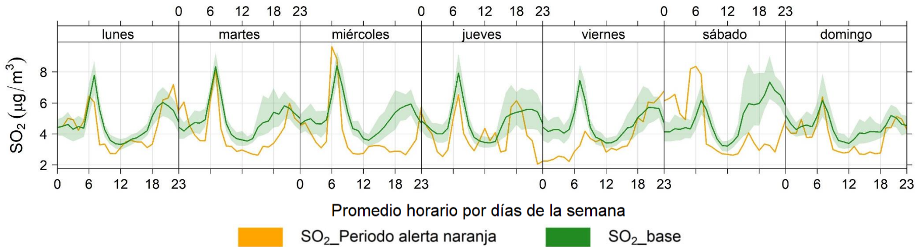
Evolución temporal de concentraciones promedio horarias por días de la semana de SO 2 durante 2023 (SO 2 _base) y su comparativo con el periodo del 7 al 13 de junio de 2023
