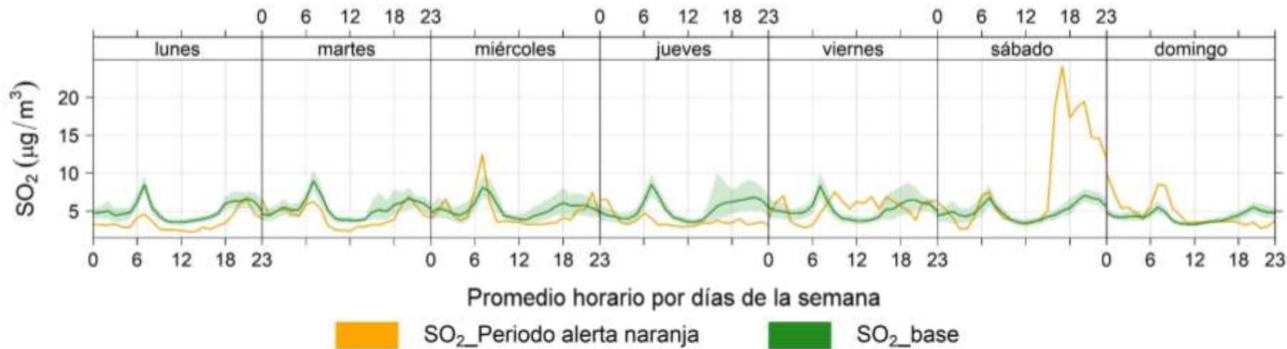
Evolución temporal de concentraciones promedio horarias por días de la semana de SO 2 durante 2023 (SO 2 _base) y su comparativo con el periodo del 19 al 25 de junio de 2023
