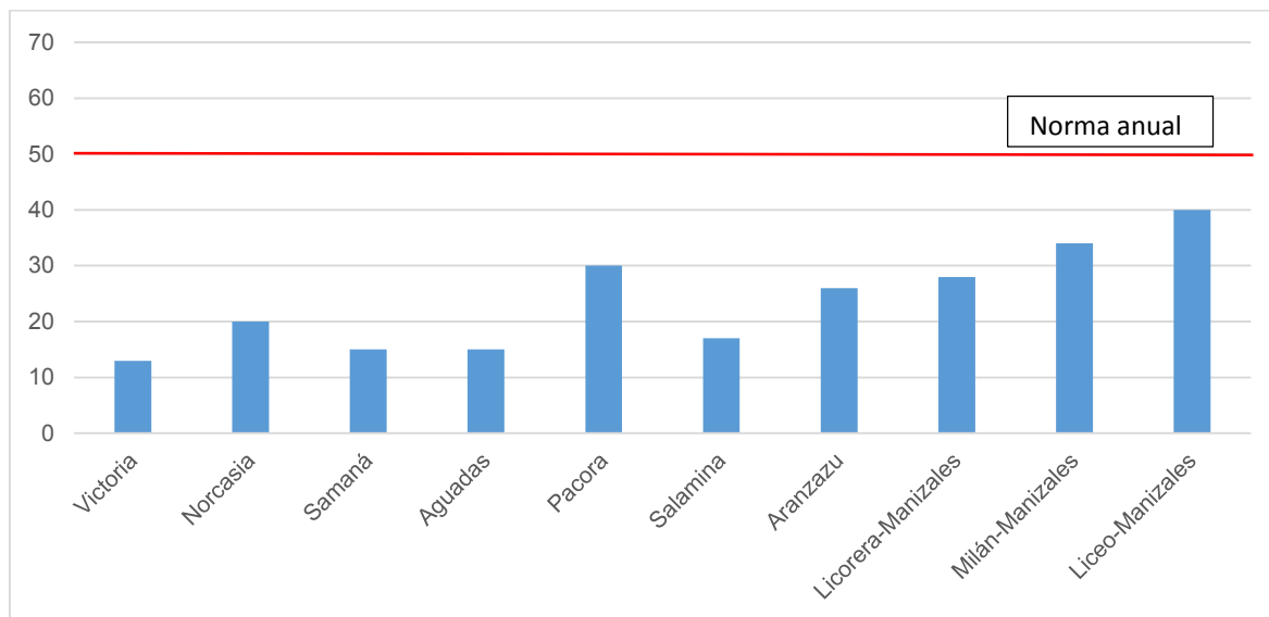
FIGURA 3: CONCENTRACIÓN DE PM 10 (µg/m 3 ) EN CALDAS.
