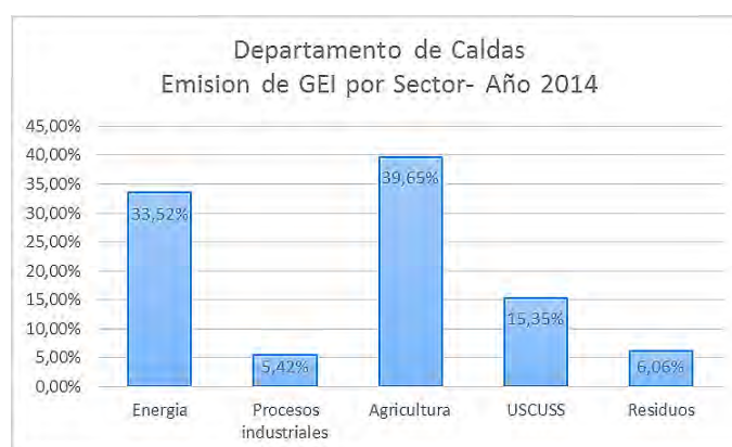
FIGURA 10: EMISIÓN DE GASES DE EFECTO INVERNADERO POR SECTOR
