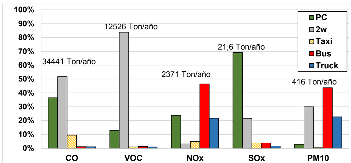
FIGURA 4: CONTRIBUCIÓN DE CONTAMINANTES POR FUENTES MÓVILES, AÑO BASE 2014.
