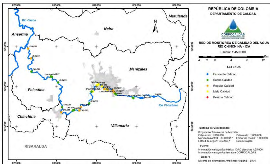
MAPA 10: ÍNDICE DE CALIDAD (ICA) DEL RÍO CHINCHINÁ, 2010.
