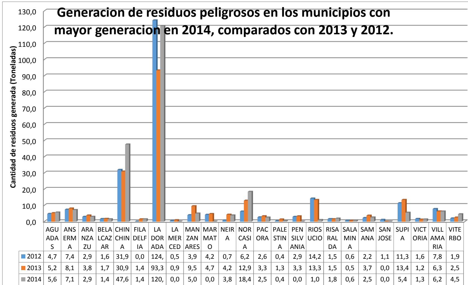
FIGURA 13: RESIDUOS PELIGROSOS EN LOS MUNICIPIOS CON MAYOR GENERACIÓN EN 2014, COMPARADOS CON 2013 Y 2012
