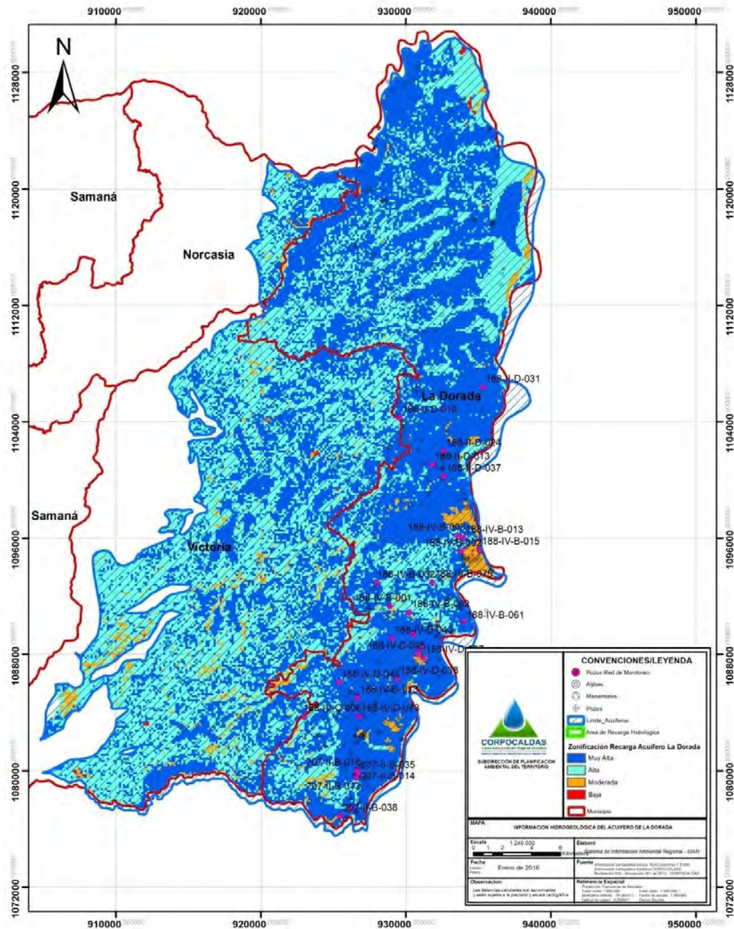
MAPA 7: INFORMACIÓN HIDROGEOLÓGICA DE ACUÍFERO DE LA DORADA
