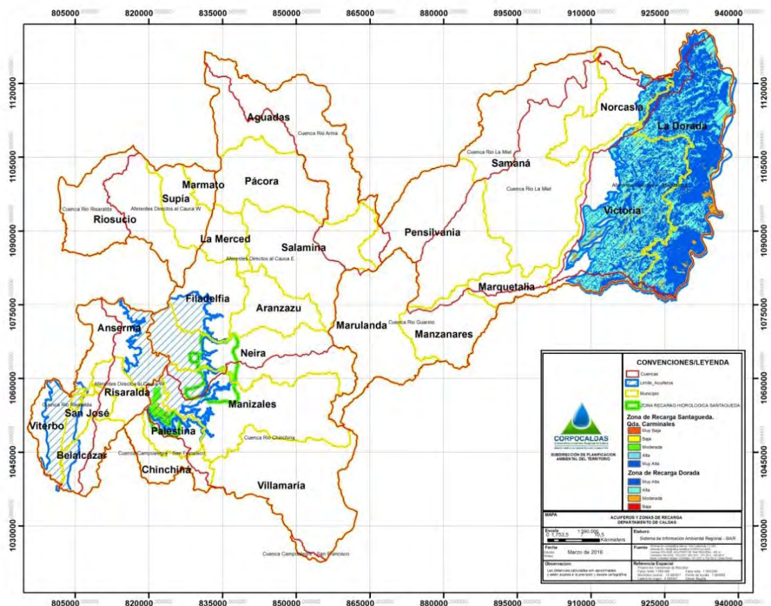
MAPA 5: ACUÍFEROS Y ZONAS DE RECARGA DEL DEPARTAMENTO DE CALDAS
