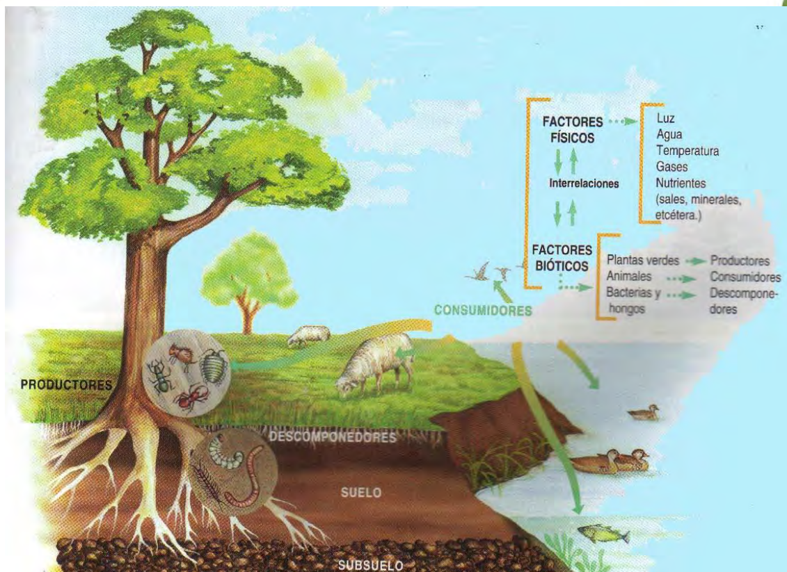
ILUSTRACIÓN 2: CICLADO DE NUTRIENTES
