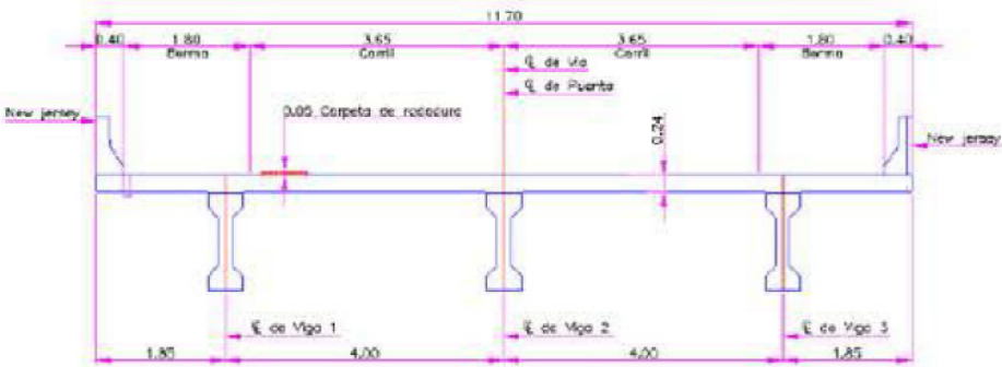
Figura 51. Sección transversal puente L = 15.0 m en la Unidad Funcional 4
