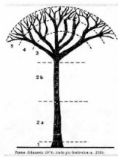
Figura 2. Estratificación de forófitos para muestreo de epífitas vasculares y no vasculares.
