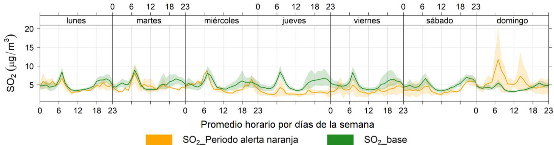
Evolución temporal de concentraciones promedio horarias por días de la semana de SO 2 durante 2023 (SO 2 _base) y su comparativo con el periodo del 31 de marzo al 16 de abril de 2023
