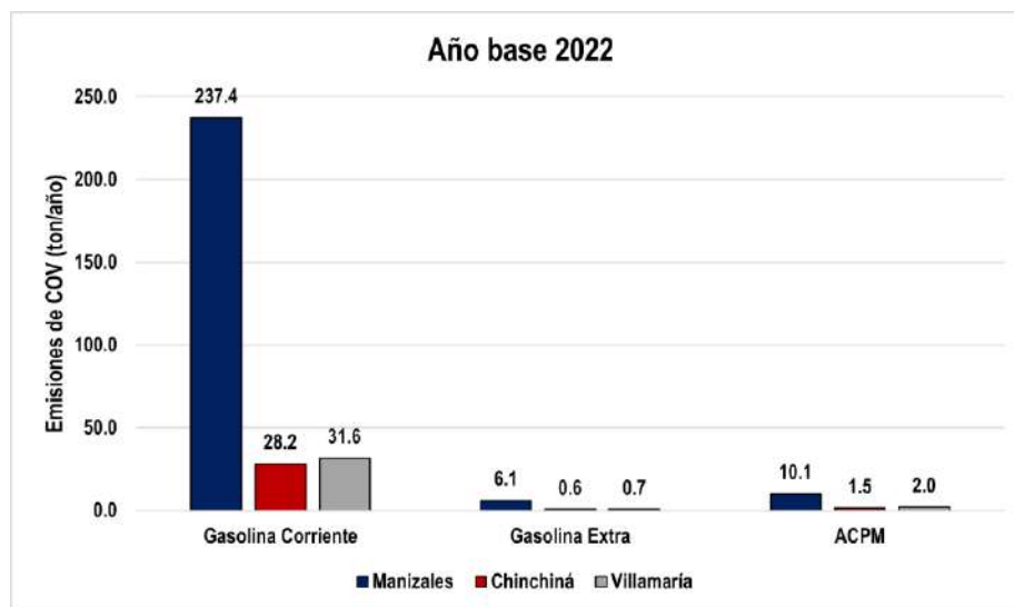
Emissiones de compuestos orgánicos volátiles- COV, 2022
