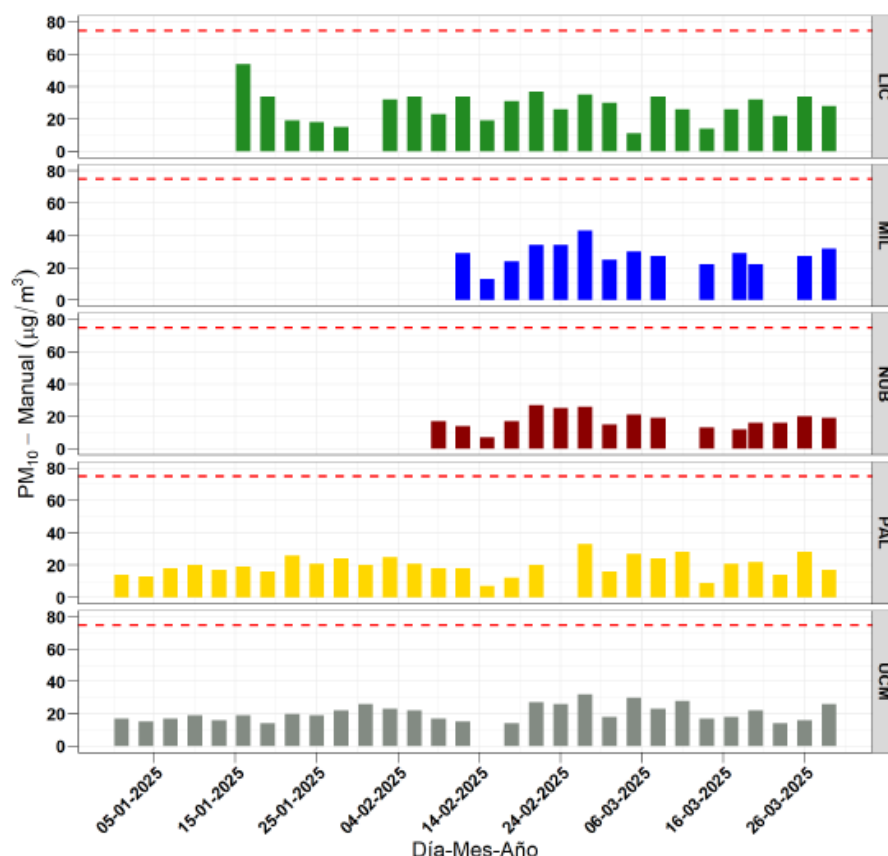
Concentraciones de PM10, estaciones Manizales, 2025
